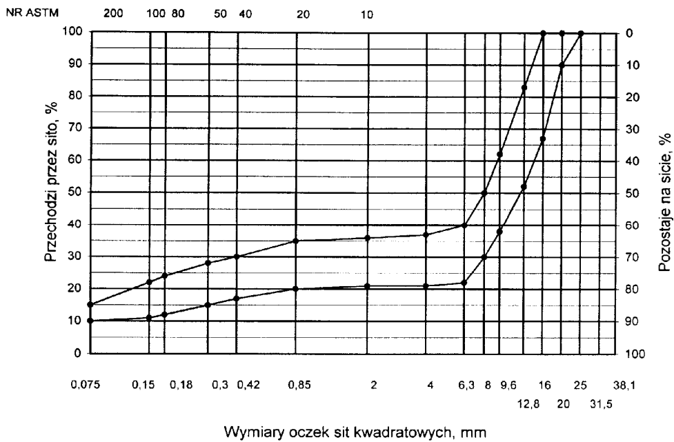
Rys. 5. Krzywe graniczne uziarnienia mieszanki mineralnej BA od 0 do 20 mm (mieszanka o nieciąglym uziarnieniu) do warstwy ściernej nawierzchni drogi o obciążeniu ruchem od KR3 do KR6
