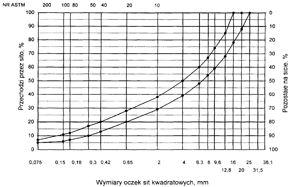
Rys. 4. Krzywe graniczne uziarnienia mieszanki mineralnej BA od 0 do 20 mm do warstwy ściernej nawierzchni drogi o obciążeniu ruchem od KR3 do KR6
