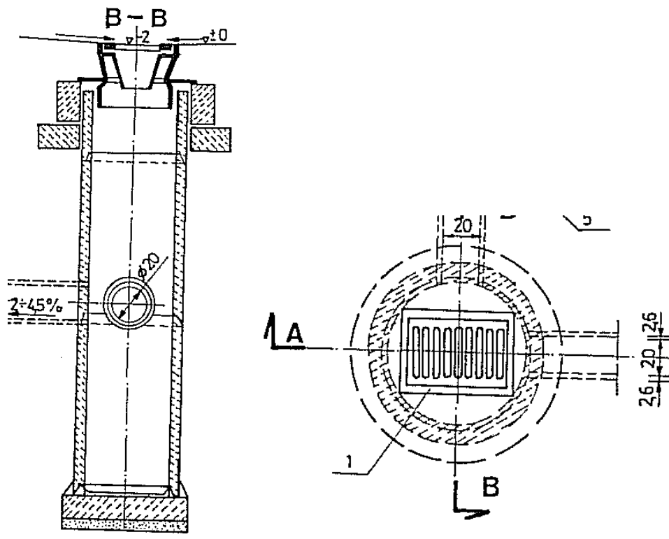
Studnie chłonne
